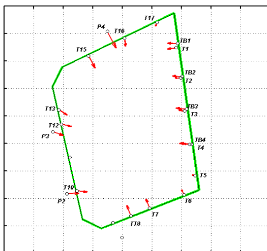
شکل ۳-۵: بردارهای جابه‌جایی نقاط نشانه مربوط به یک پروژه گودبرداری
