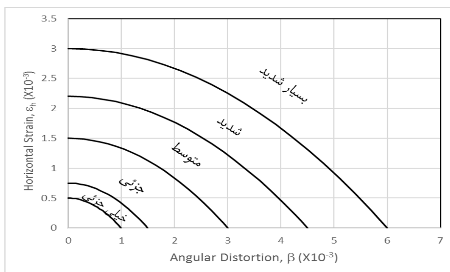
شکل ۳-۲: نمودار معیار آسیب دیدگی سازه ها براساس مقدار جابه جایی نسبی فونداسیون ها
