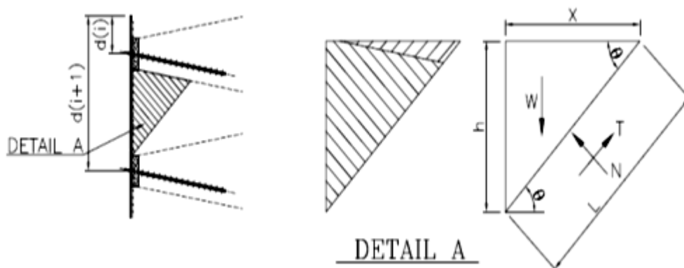
شکل ۱-۳: بلوک لغزشی فرضی بین دو ردیف مهار و دیاگرام آزاد نیروهای وارد بر آن
